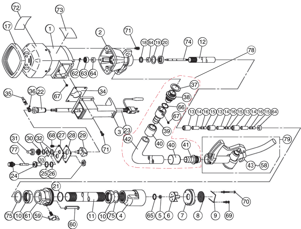
型式名 FA-100-AAA-1 (004851022)
