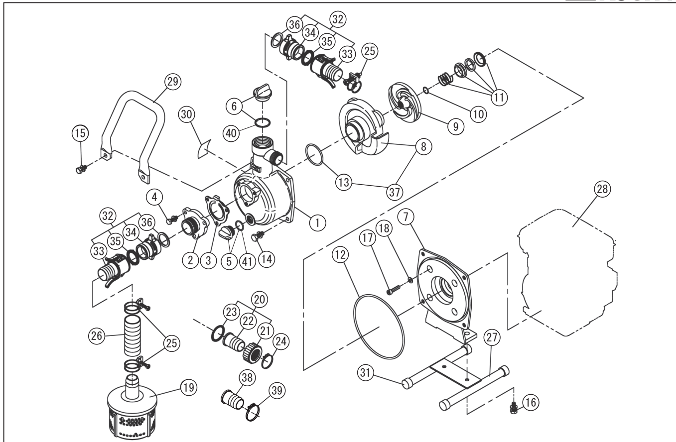
型式名 KH-25 (SEH-25L-AAA-0) &lt;GX25&gt; (012879905)
