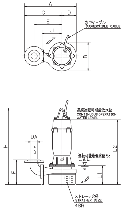
吐出し曲管分割形
